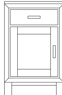
1 adj shelf 20x18x32 37-1981-__
