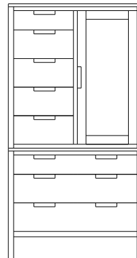
2 adj shelves 35x18x62 31-1713-__
